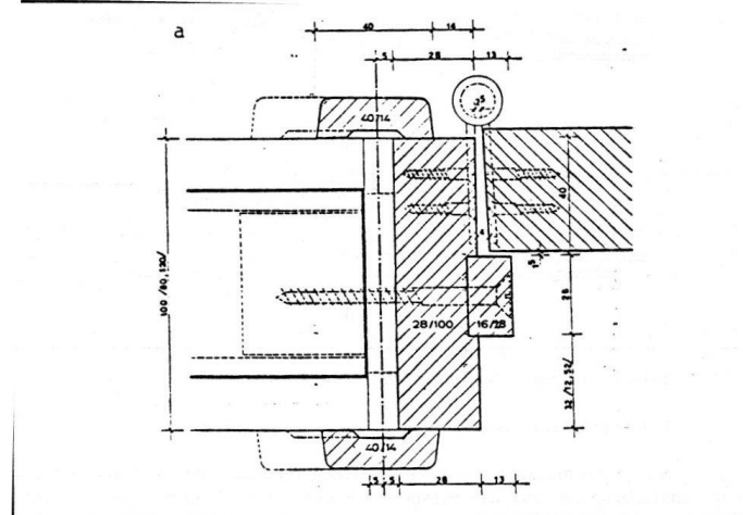
Slika 1.1.36. Vrata vrste S
