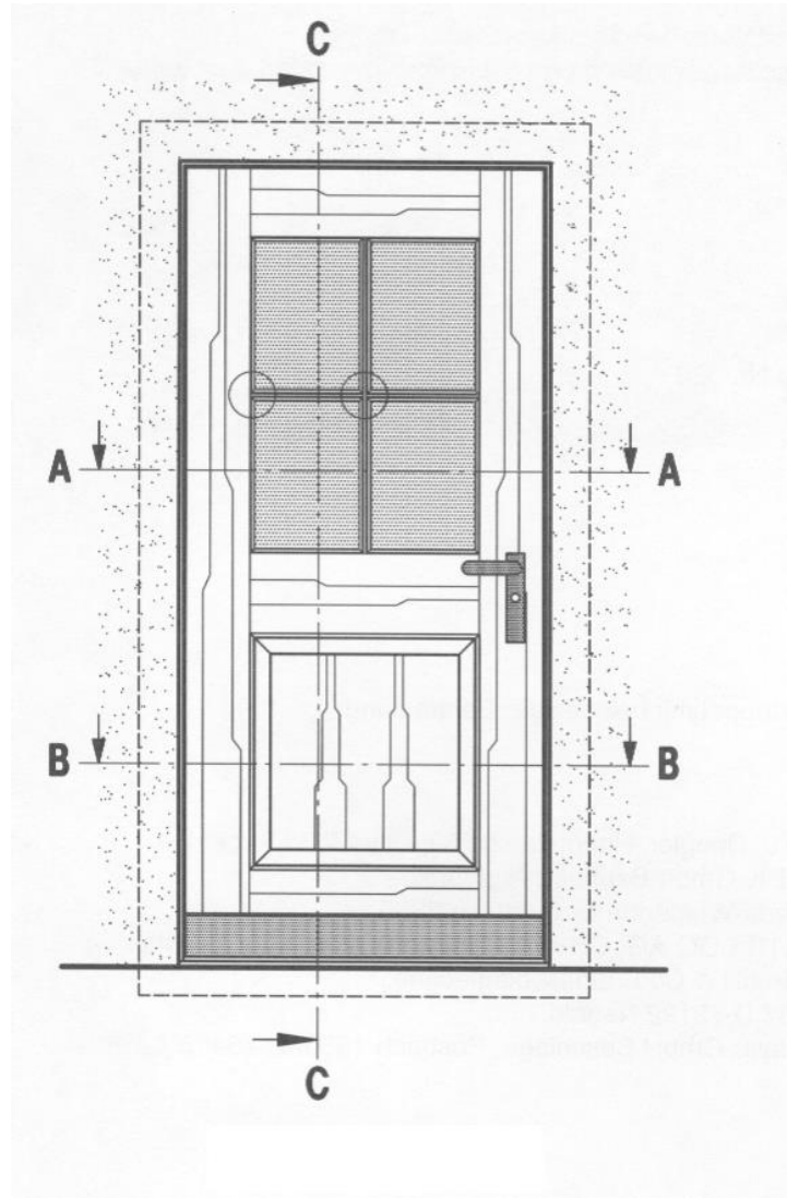
delimično zastakljena vrata
