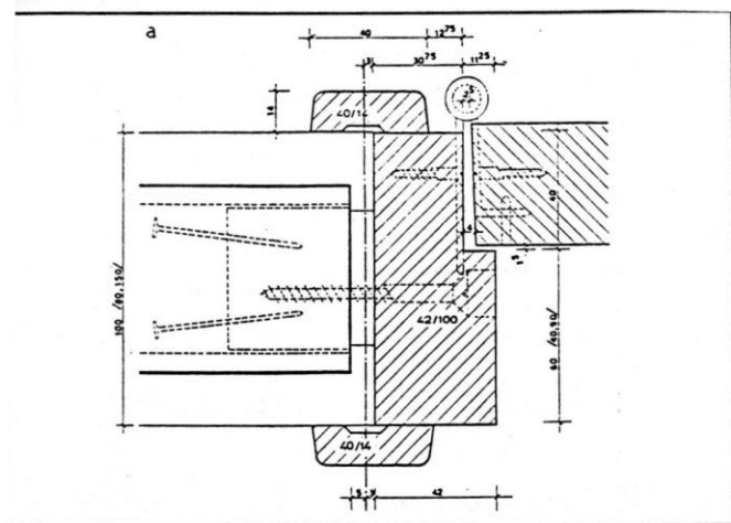
Slika 1.1.35. Vrata vrste R
