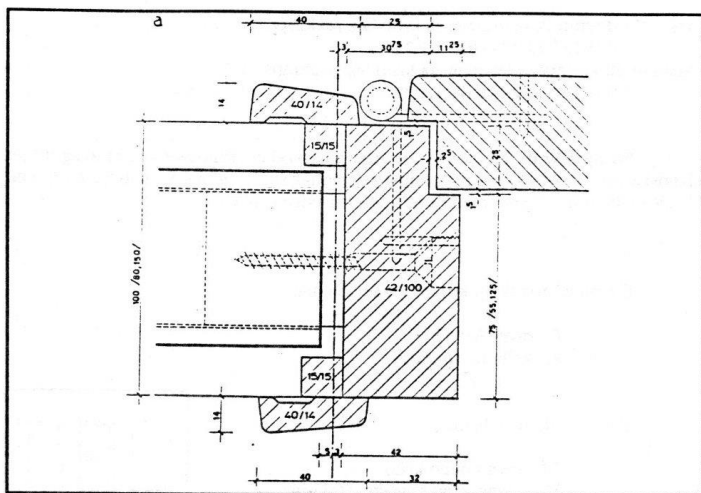
Slika 1.1.33. Vrata vrste M
