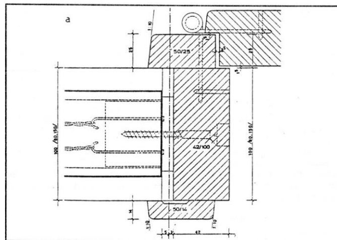
Slika 1.1.34. Vrata vrste N
